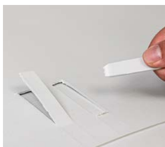
Schältest (2 cm mit Abriss außerhalb der Fügenaht)
